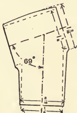
Fig. 19.—Lower Horizontal Lug.
